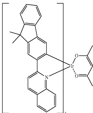
Ir(Flq) 2 (acac)
